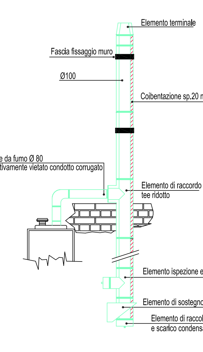
PARTICOLARE INSTALLAZIONE GENERATORE MURALE
