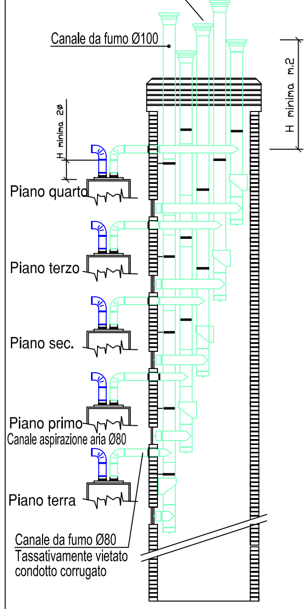
INSTALLAZIONE IN CAVEOIO - COPPELLA COIBENTE ACCIAIO INOX PARETE SEMPLICE Ø100 mm.
