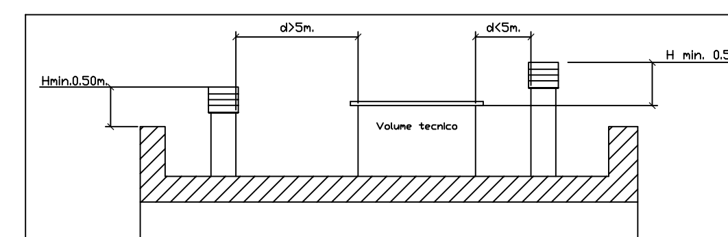
PARTICOLARE INSTALLAZIONE GENERATORE MURALE
